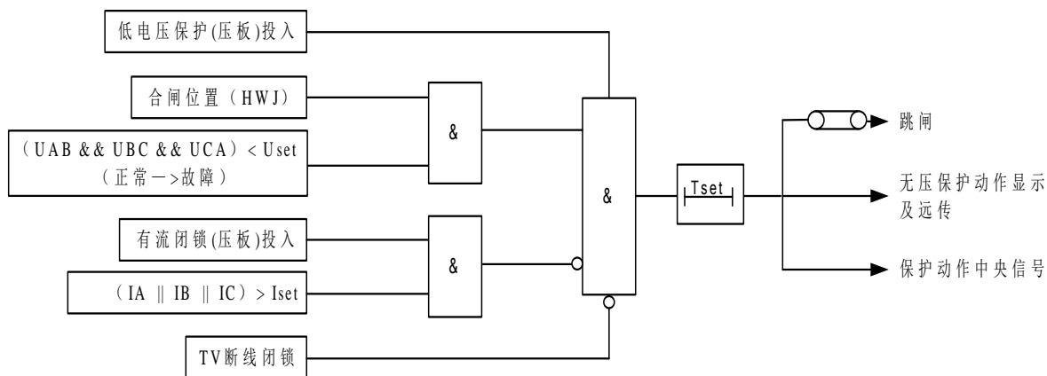
图 13 低电压保护逻辑图
