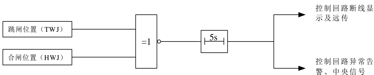
图 16 控制回路断线逻辑图
