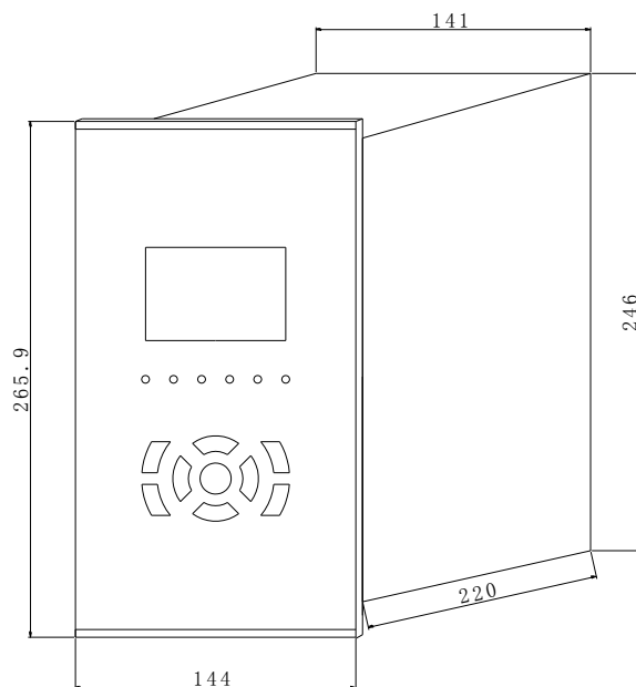
图 3 NZB7121/NZB7122/NZB7123/NZB7128 产品外形尺寸图
