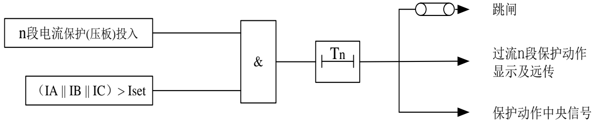
图 9 定时限过流保护逻辑图
