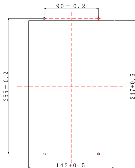
图 4 NZB7121/NZB7122/NZB7123/NZB7128 产品开孔尺寸图
