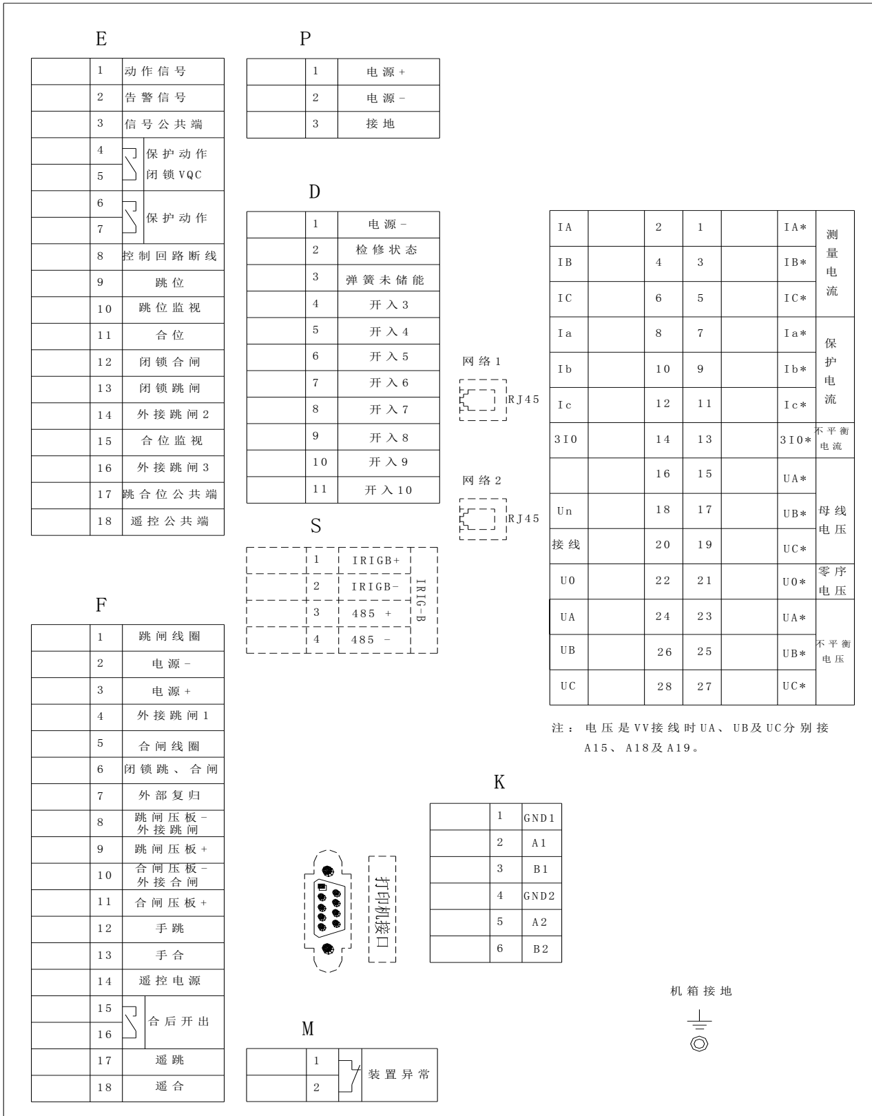
图6 NZB7128DC/AC端子图
