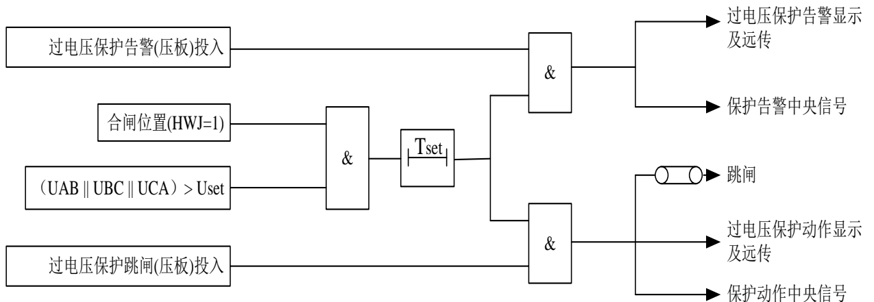
图 12 过电压保护逻辑图
