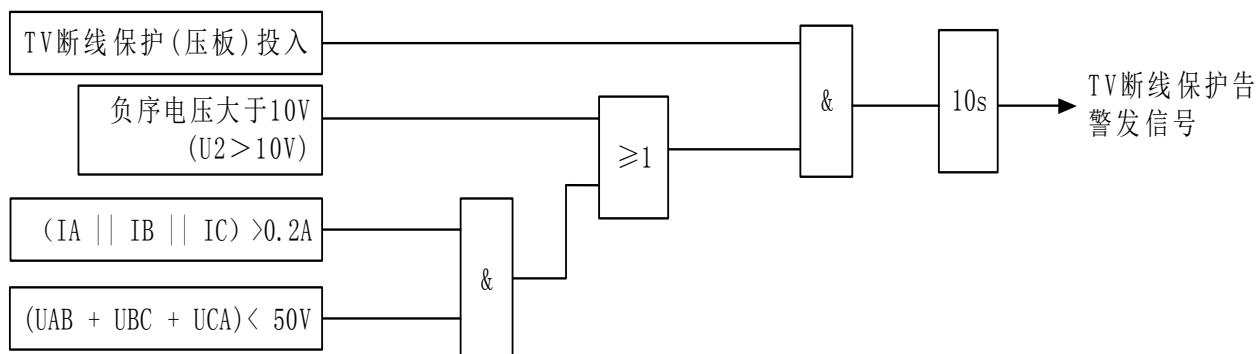
图 15 TV 断线逻辑图
