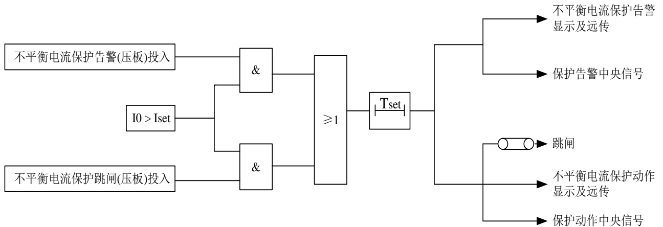
图 10 不平衡电流保护逻辑图
