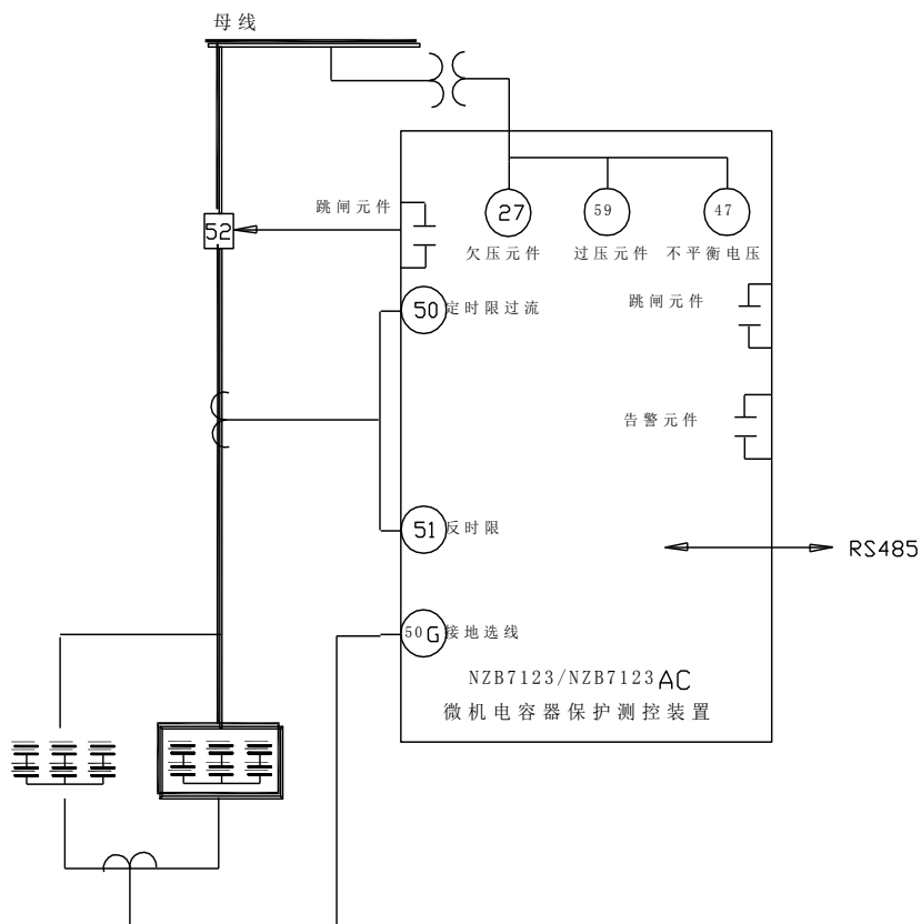
图 2 NZB7123/NZB7123AC 功能配置图
