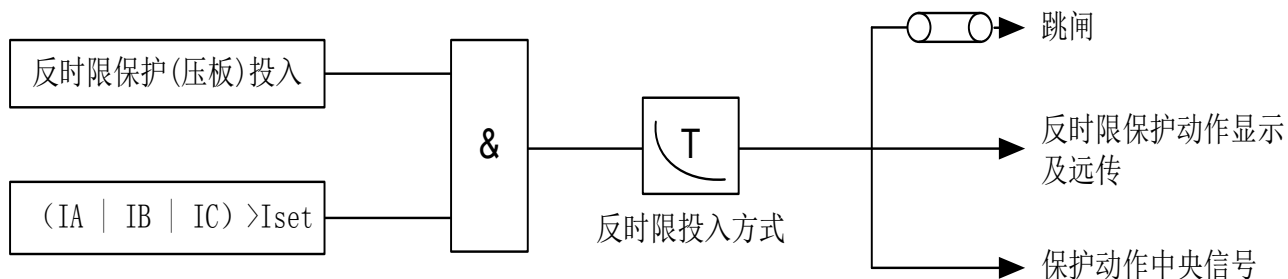
图 14 反时限保护逻辑图
